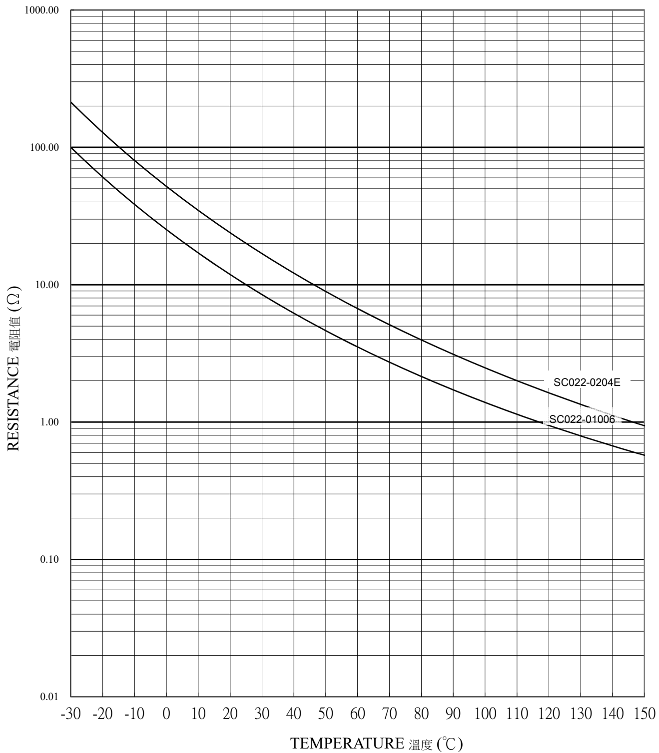
SC022 R-T CURVE 電阻-溫度曲線
