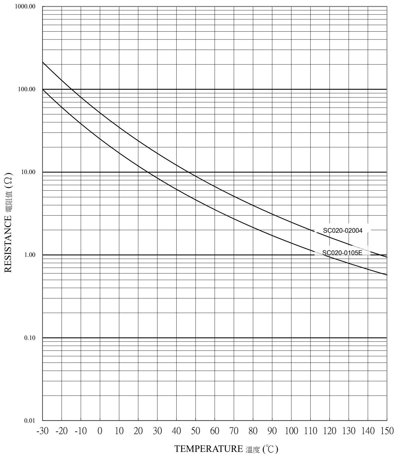
SC020 R-T CURVE 電阻-溫度曲線
