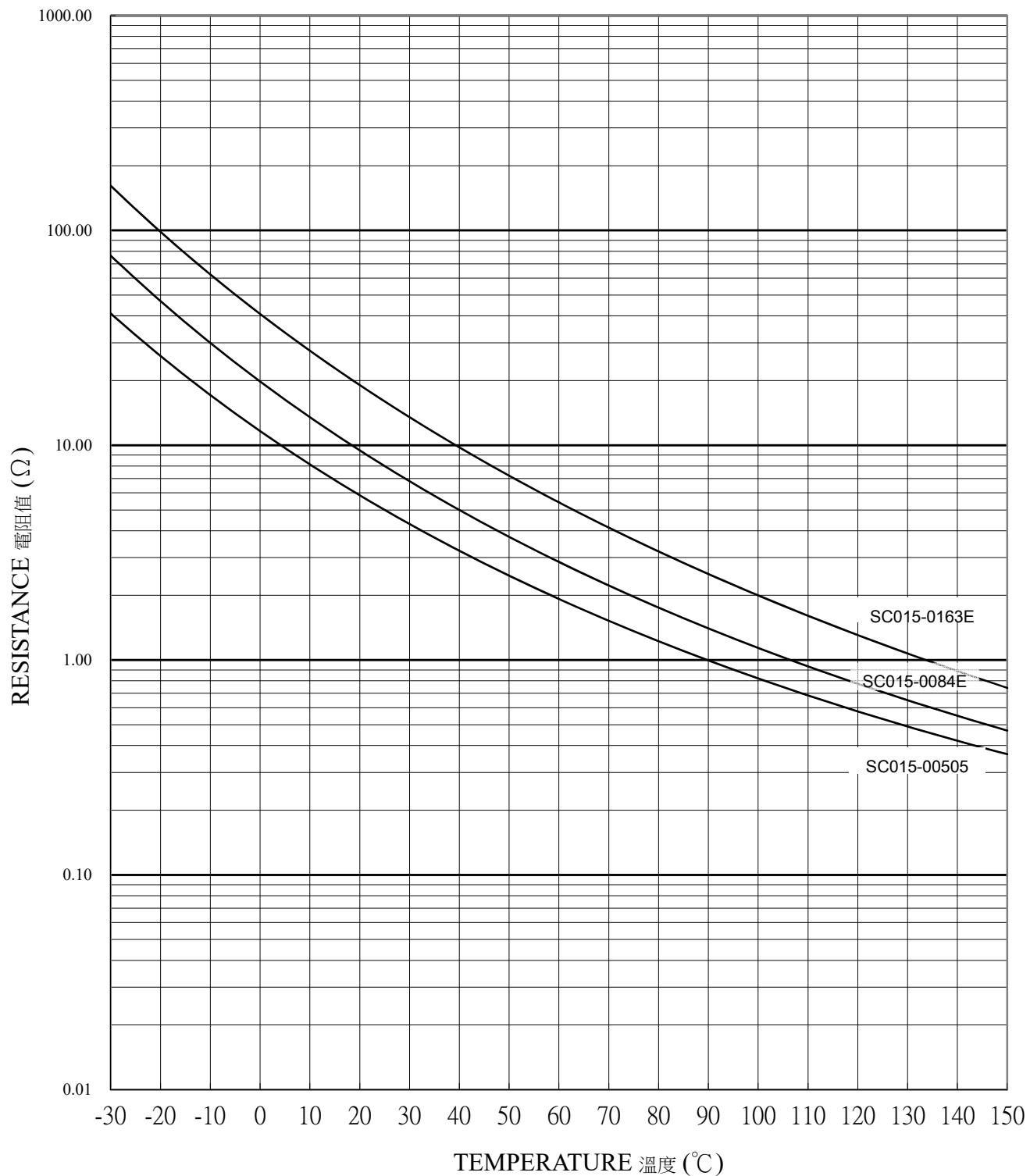
SC015 R-T CURVE 電阻-溫度曲線
