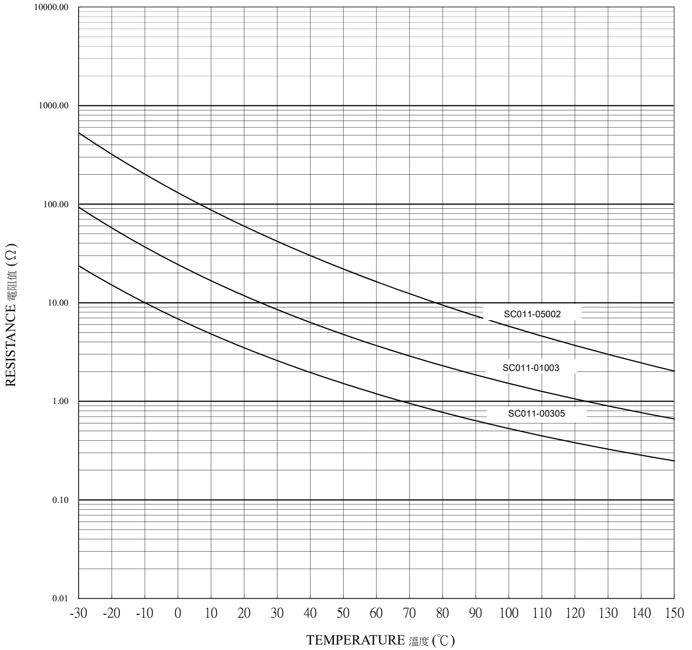
SC011 R-T CURVE 電阻-溫度曲線
