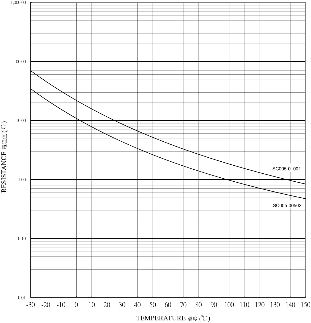
SC005 R-T CURVE 電阻-溫度曲線
